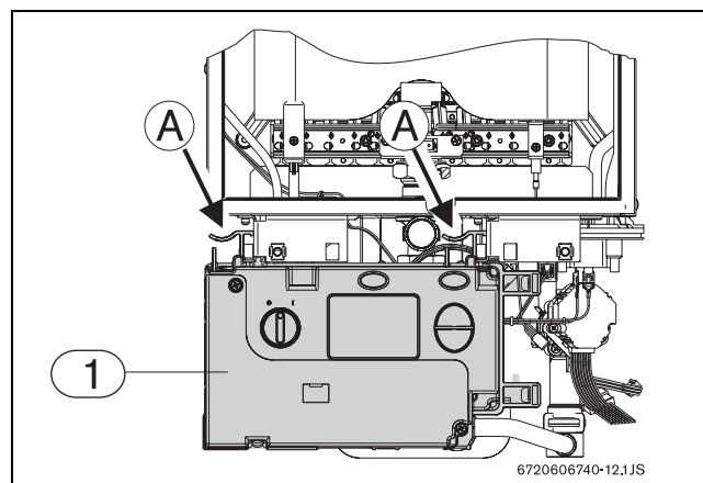
Fig. 17 Estrarre il quadro comandi
