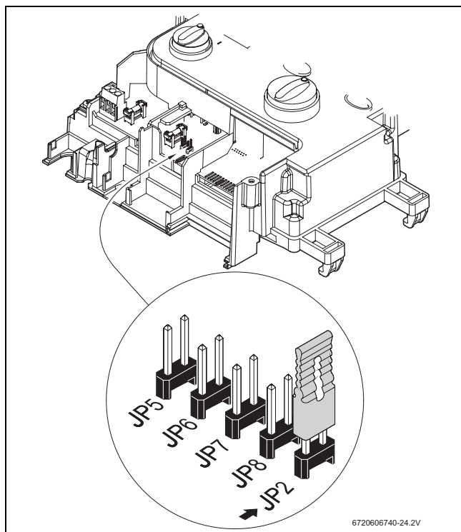
Fig. 27 Inserimento del ponticello JP2
