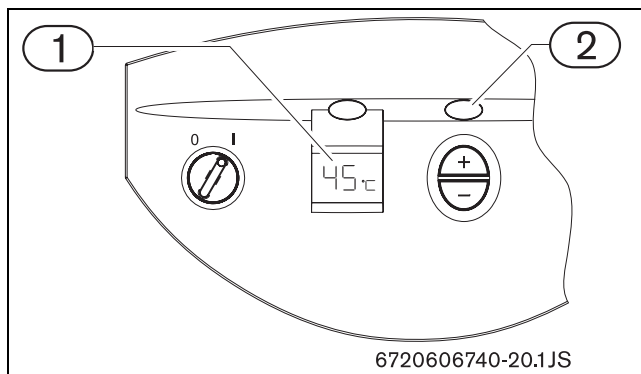
Fig. 8 Quadro comandi
