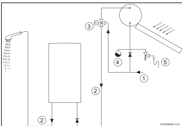
Fig. 12 Impianti solari
