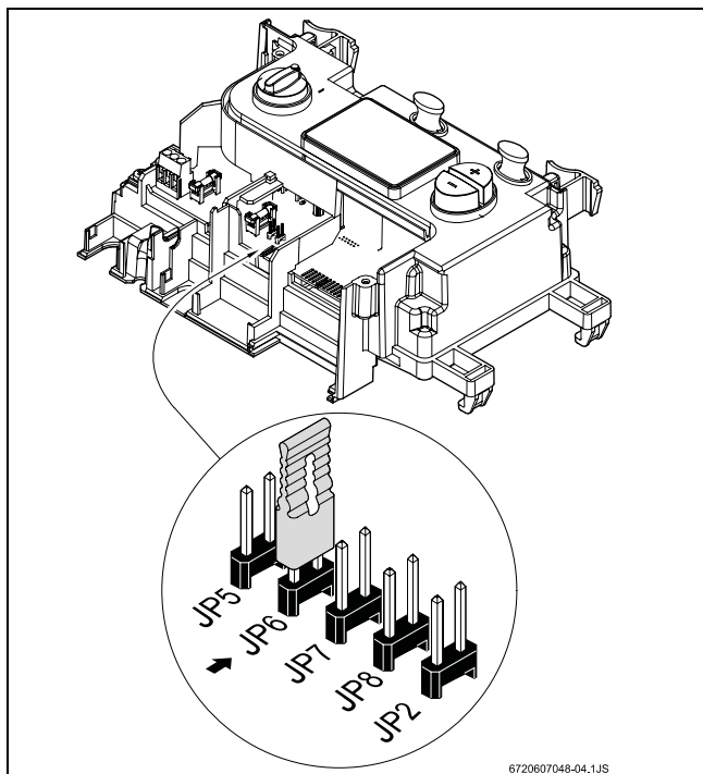
Fig. 24 Posizione morsetti e ponticello
