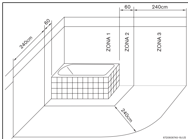
Fig. 13 Raffigurazione della Zona 3 (CEI 64-8)
